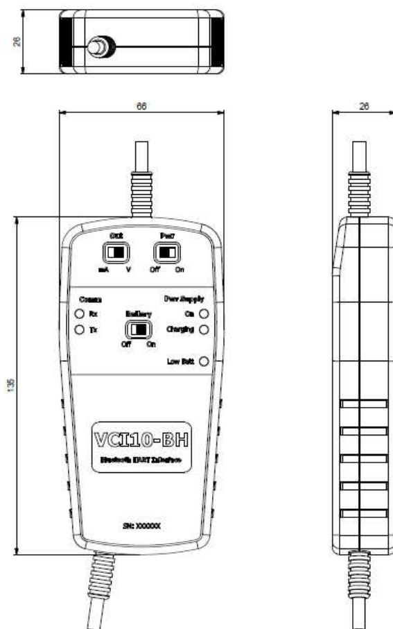
Figura 7.1 – Dimensiones mecánicas de la VC110-BH.
